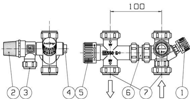
ЛК-КЛАПАННАЯ ГРУППА Д 22/18
